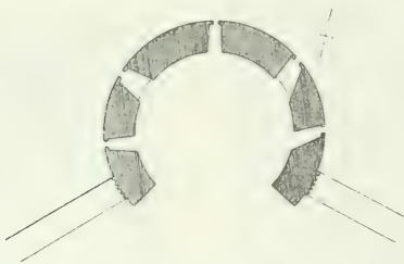
Grundriss af «Hanetaarnet» med tilstødende Plankebefæstning.
